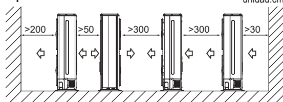
Conexión paralela de los frentes y partes traseras
