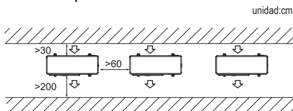
Conexión en paralelo dos unidades o más
